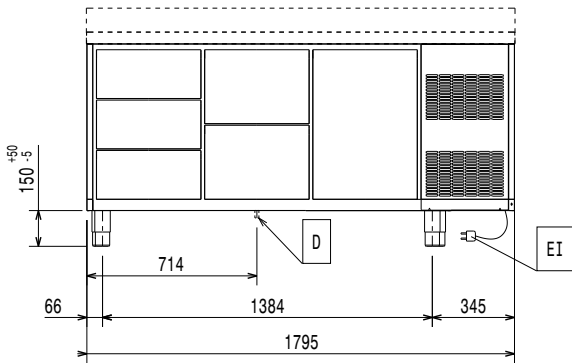
Front aanzicht
